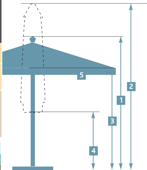
Modèle hors standard : toile orchestra SANS LAMBREQUIN
